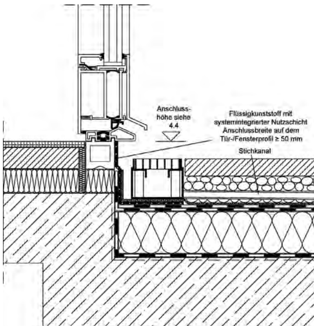
Terrassentüranschluss mit Entwässerungsrinne - Anschlusshöhe \geq 5 cm - Ausführung mit Flüssigkunststoff (im Anschlussbereich mit systemintegrierter Nutzschicht)
