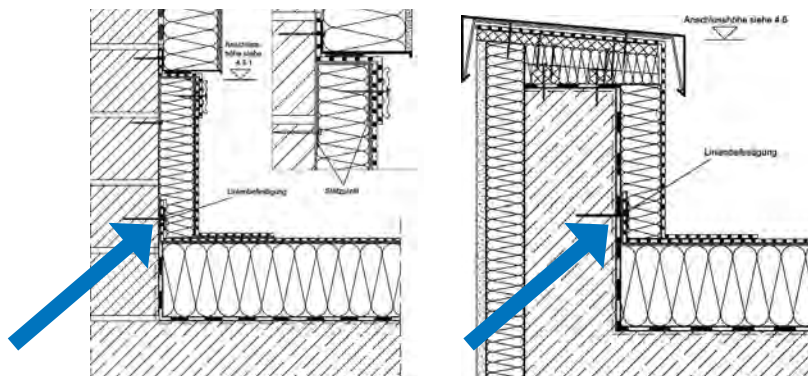
Beispielhafte Details für eine Randfixierung bei Kunststoffbahnen
