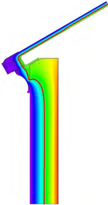
Querschnitt Basisprofil
